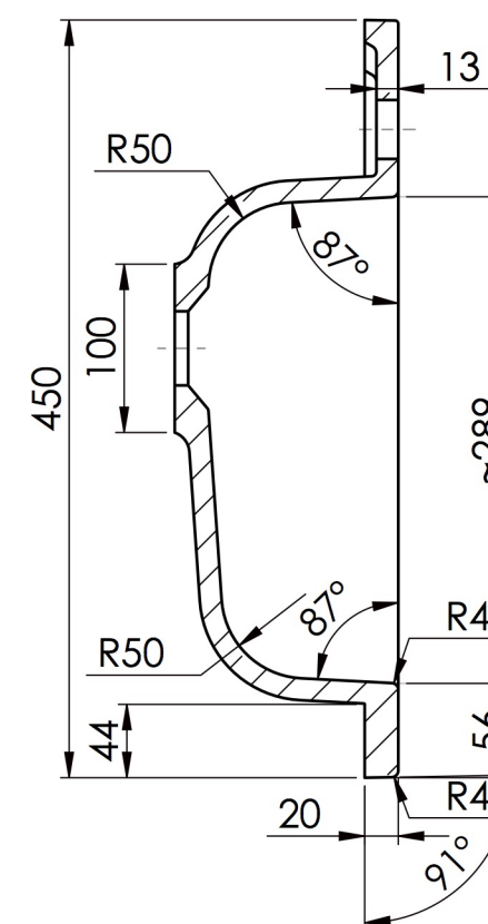
B-B (1 : 5)
