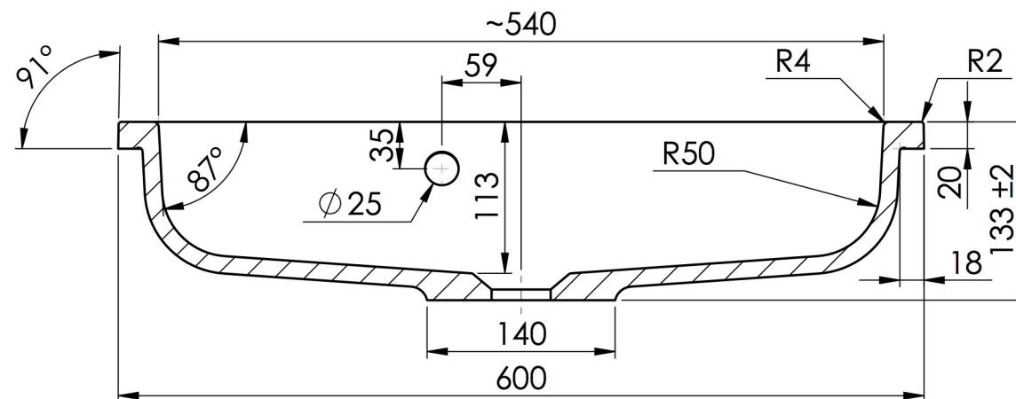
A-A (1 : 5)
