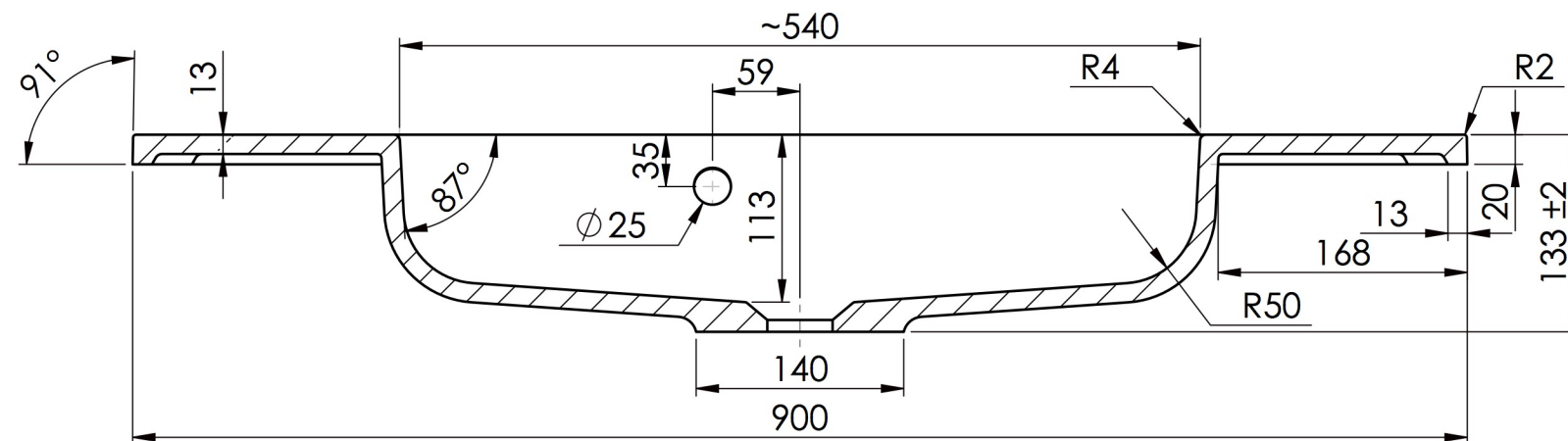
A-A (1 : 5)
