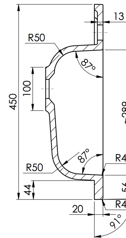
B-B (1 : 5)
